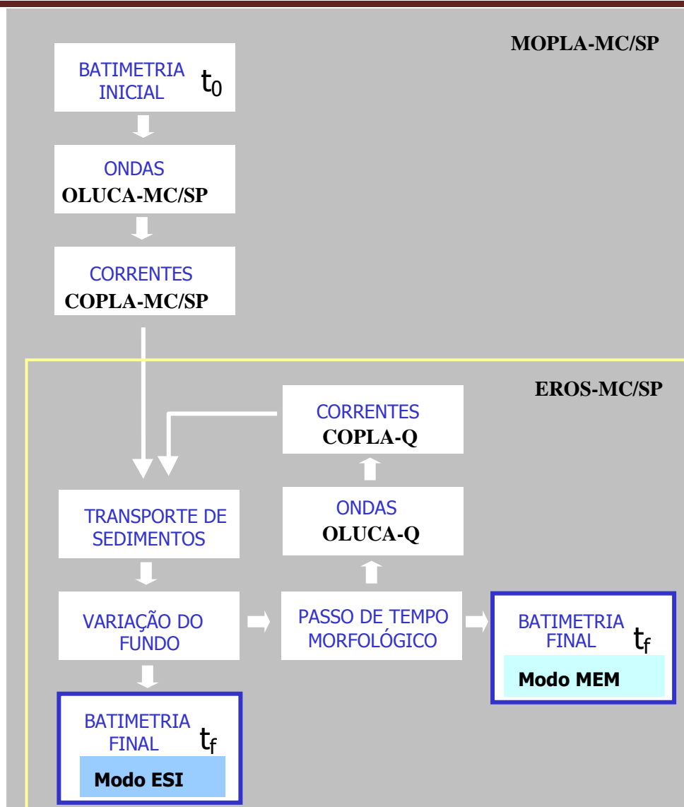
Figura 2 – Estrutura EROS.
