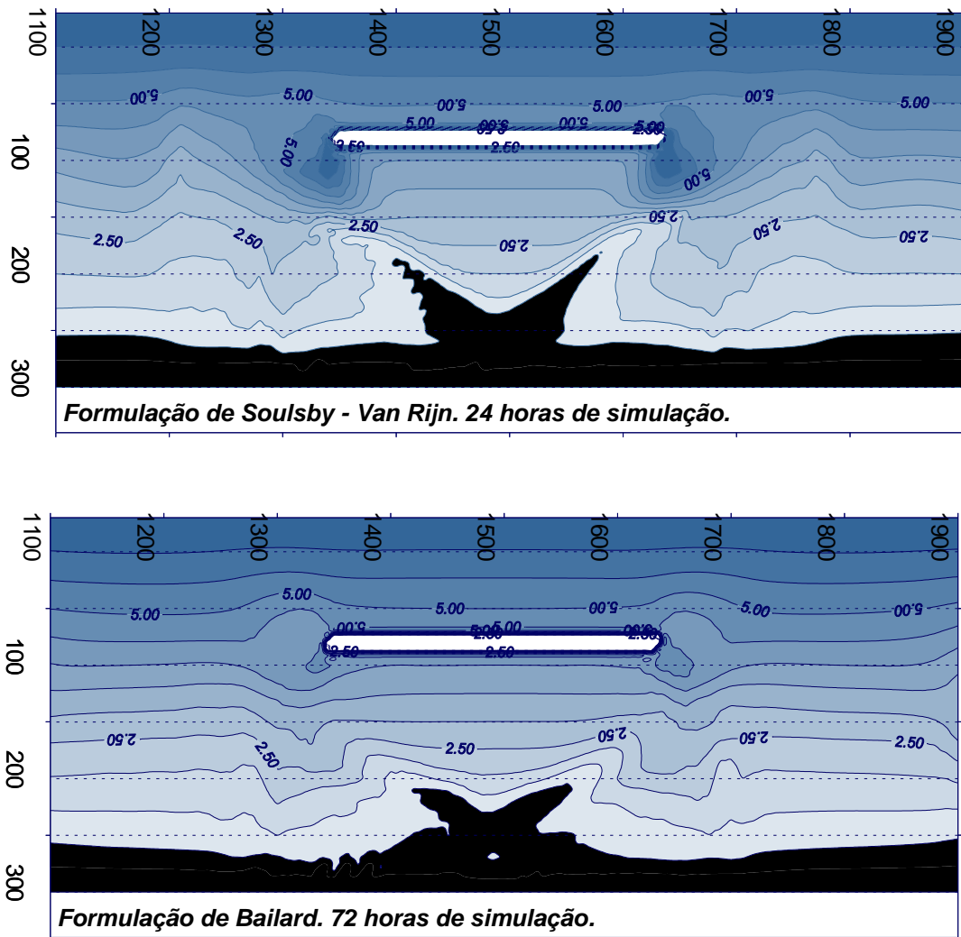
Figura 7 – Resultados do EROS-MC, baseado na formulação de Soulsby – Van Rijn (24h) e Bailard (72h).
