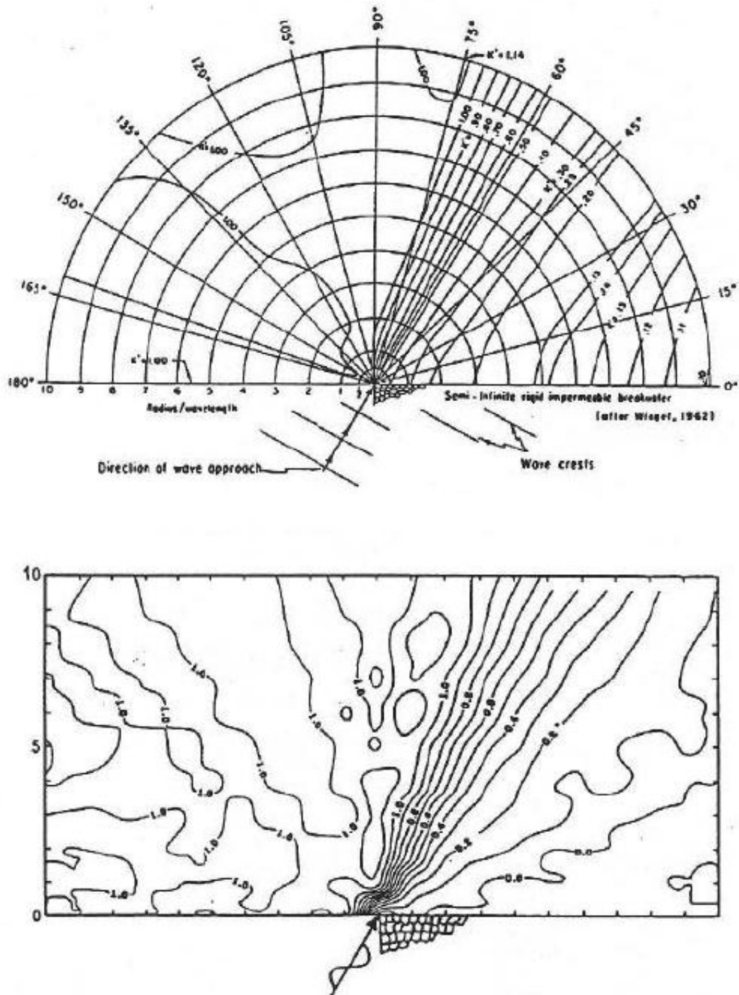
Figura 18 – Diagrama de difração das ondas. Comparação com a solução analítica. Ângulo de incidência: -30^\circ .
