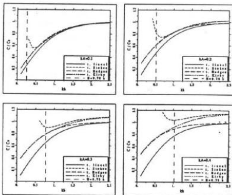
Figura 1 – Variação das relações de dispersão lineares e não lineares com kh e esbeltez da onda \epsilon (KIRBY; DALRYMPLE, 1986 a).
