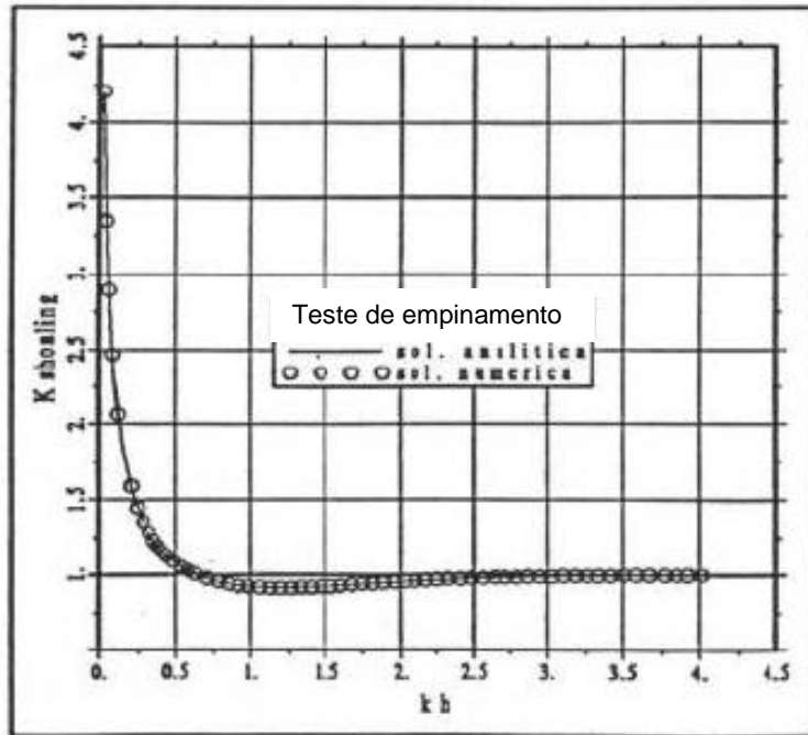
Figura 15 – Fenômeno de empinamento sobre uma declividade.
